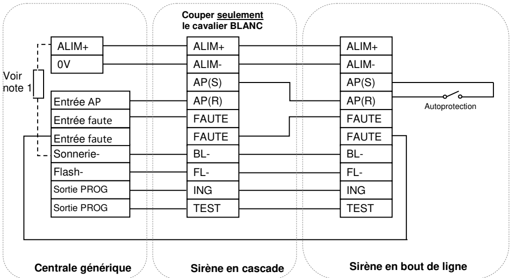
Fig. 2 : Branchement auto-protection MAGNA-F (multiple en cascade)
